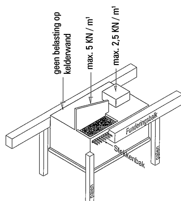
3 Kelder aan funderingsbalk opgehangen
