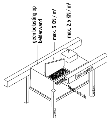
1 Kelder aan funderingsbalk opgehangen
